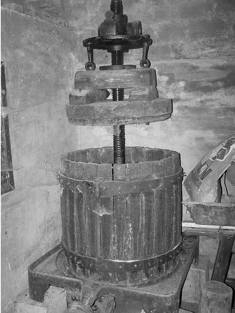
Txakolina egiteko dolarea, 2008.
