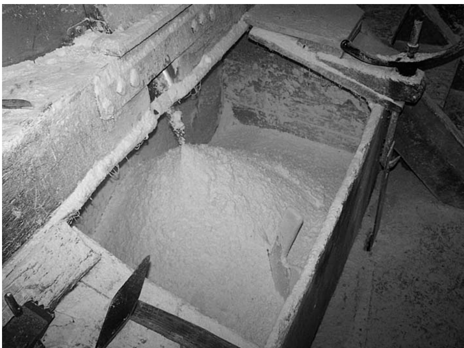
Ehotzea amaitzen denean irina urun-askara jausten da, 2008.
